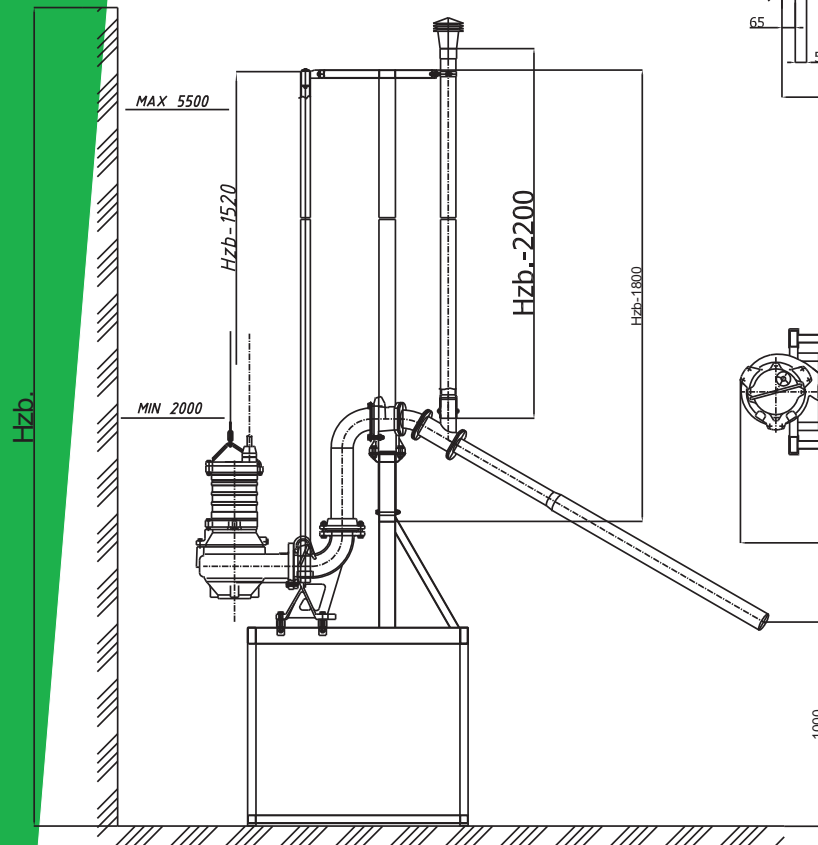
Strumienica S2S-44ZN;-54ZN; -74ZN; -94ZN; -114ZN
